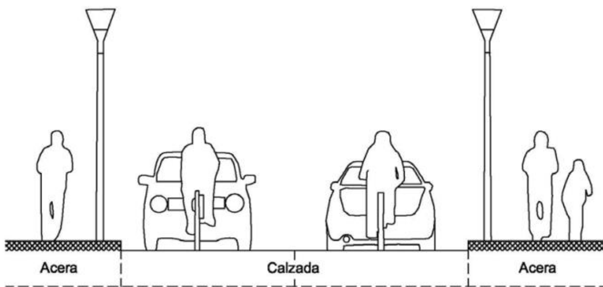
Figura 2. Sección ciclocalle.
