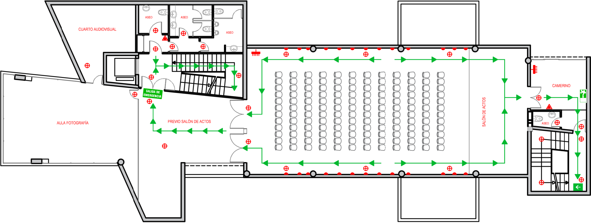
PLANTA NIVEL +1
