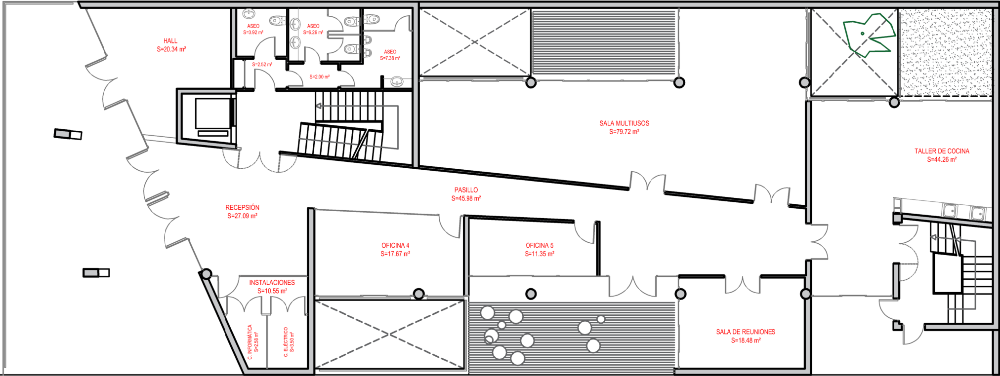
PLANTA NIVEL ±0
