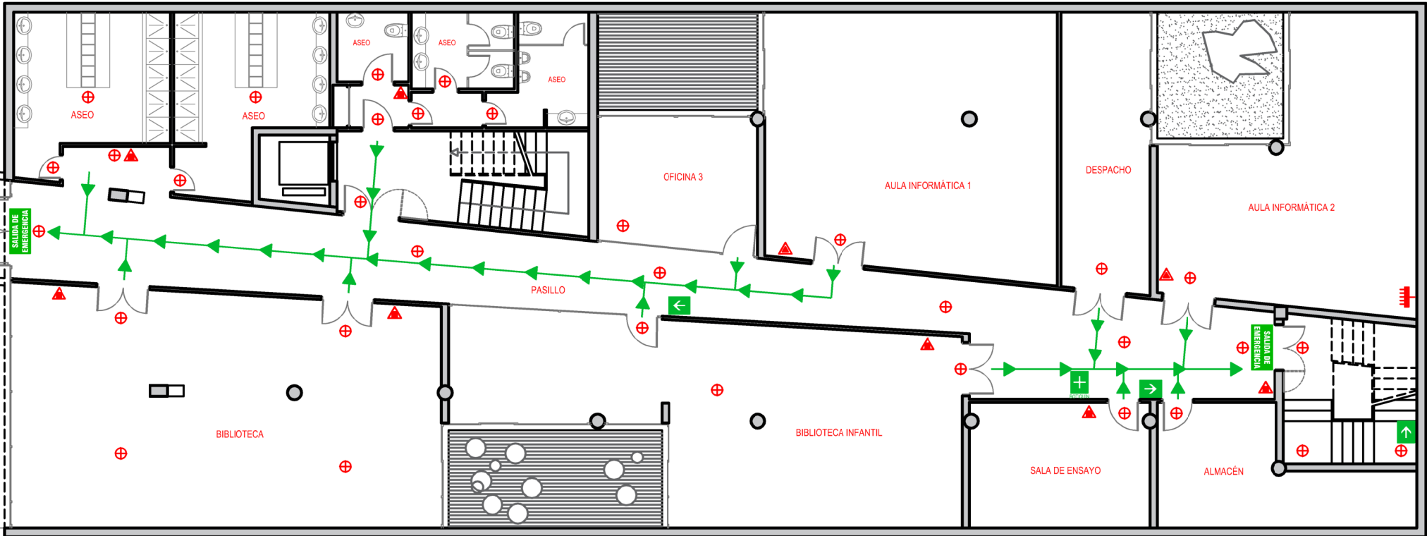
PLANTA NIVEL -1
