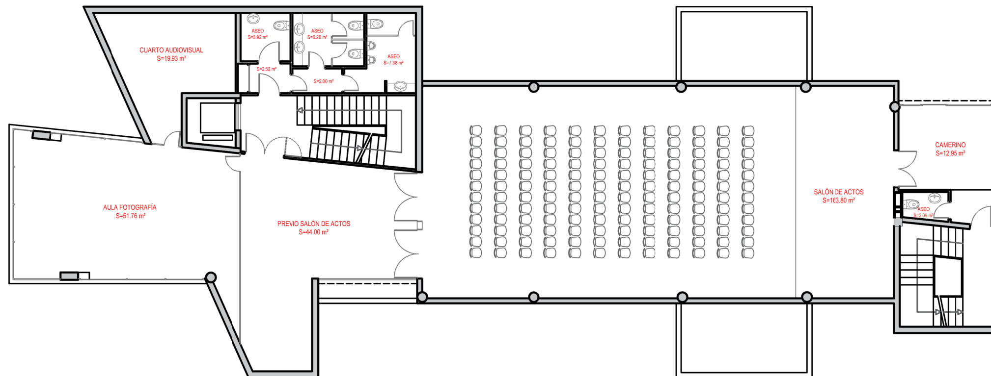
PLANTA NIVEL +1
